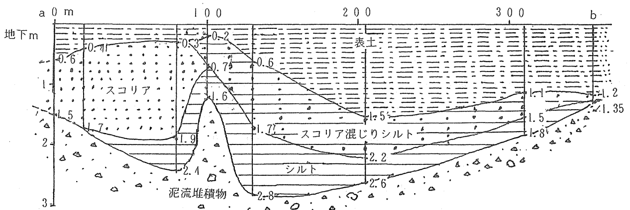
図1. 古大胡田湖の断面 a-b.
