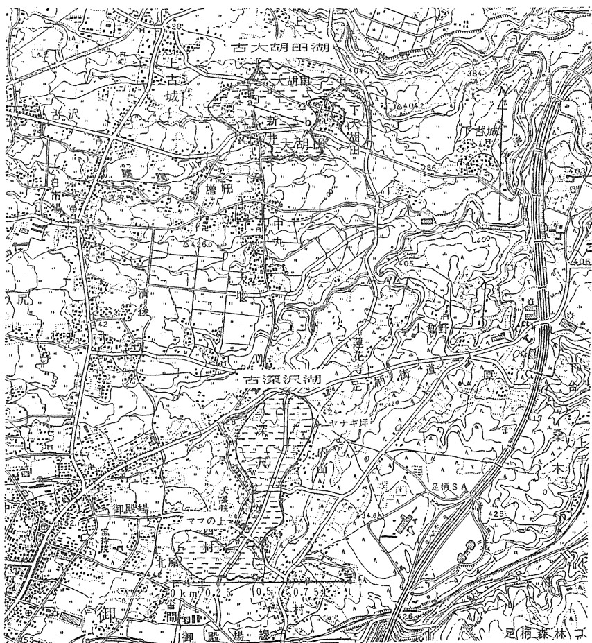
図2. 古大胡田湖, 古深沢湖.
