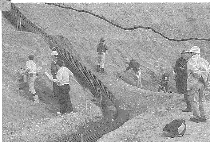
写真2 空港ターミナル予定地点の露頭観察 黒線は相良層群切山泥岩優勢互層(下部)と坂部原礫層(上部)との境界(不整合)
