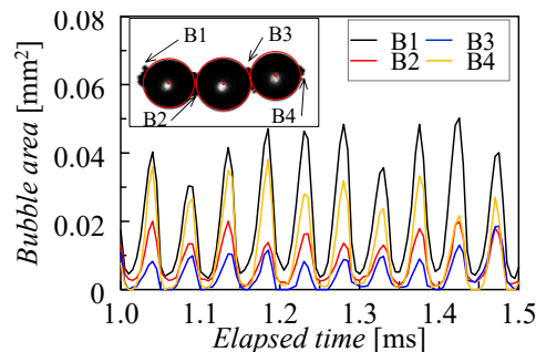
図10 粒子凝集体に付着したキャビテーション気泡の振動特性 (GC4)
