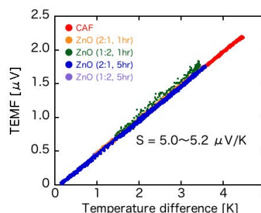
図2 炭素布上のZnOナノ結晶とゼーベック係数測定結果
