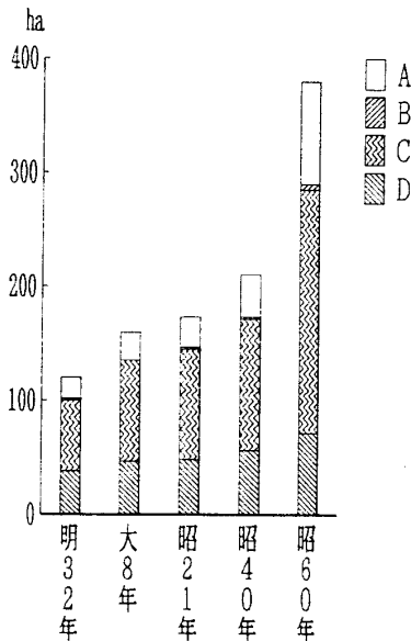
図11. 軟弱地盤地帯の市街化面積 ③ 三島駅より3～5 km A, B, C, Dは軟弱地盤のA層, B層, C層, D層に対応する。単位はha
