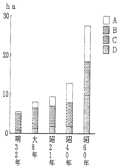
図10. 軟弱地盤地帯の市街化面積 ② 三島駅より3 km以内 A, B, C, Dは軟弱地盤のA層, B層, C層, D層に対応する。単位はha
