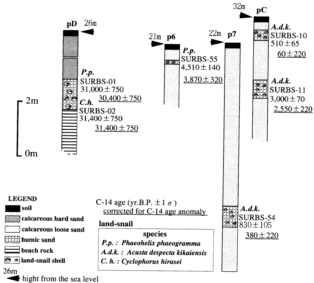
図6 喜界島の風成砂丘地質柱状図と化石陸産貝類の 14 C年代と補正年代
