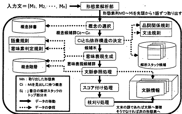
図2 構文・意味解析の処理の流れ
