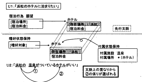
図5 構造的曖昧性を解消する例
