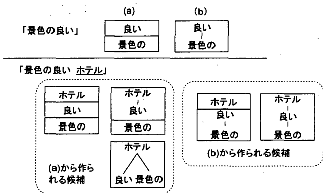
図3 「景色の良いホテル」の解析過程
