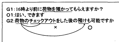
図6 文脈の情報から解析が成功する例
