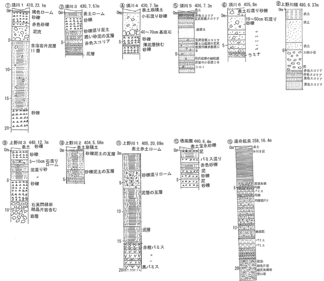
図2 扇状地(水成)堆積地層柱状図
