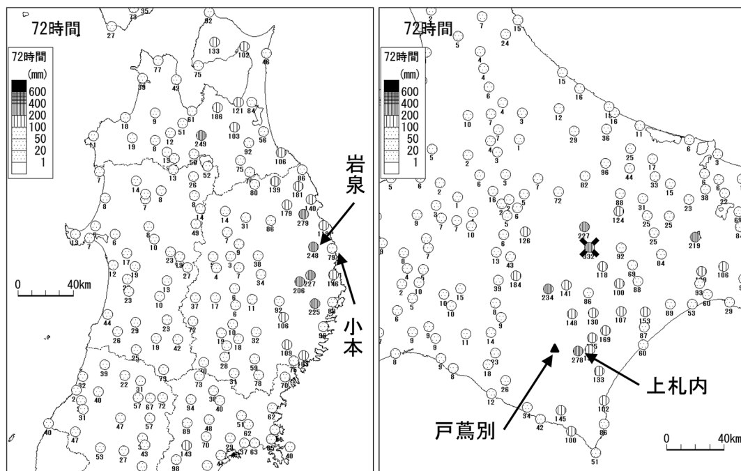
図3 8月31日24時の72時間降水量の分布。×は観測史上最大値を更新。戸蔭別は位置のみを表記した。
