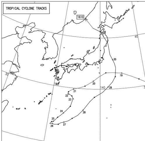
図1 台風10号の経路図(気象庁ホームページより)
