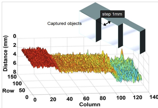
図 2 サブ mm 分解能での 3 次元形状計測。
