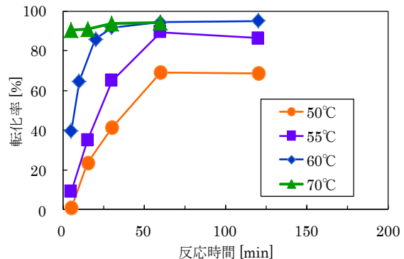
図 2 ポリ乳酸への転化率の反応温度及び反応時間依存性 (10 MPa、20wt/vol% L-ラクチド、0.5wt% DBU 触媒)
