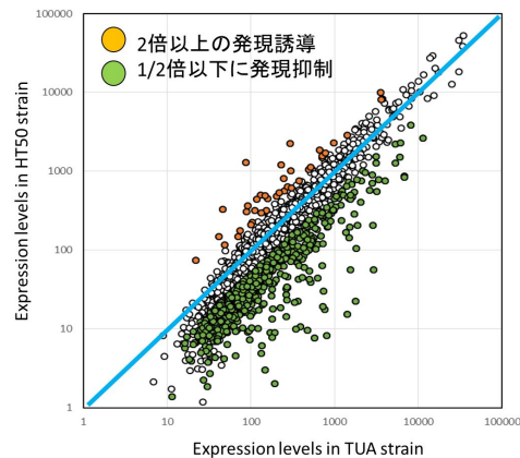
図 1. 転写産物レベルでの TUA 株と高温耐性突然変異株 (HT50 株) の比較結果
