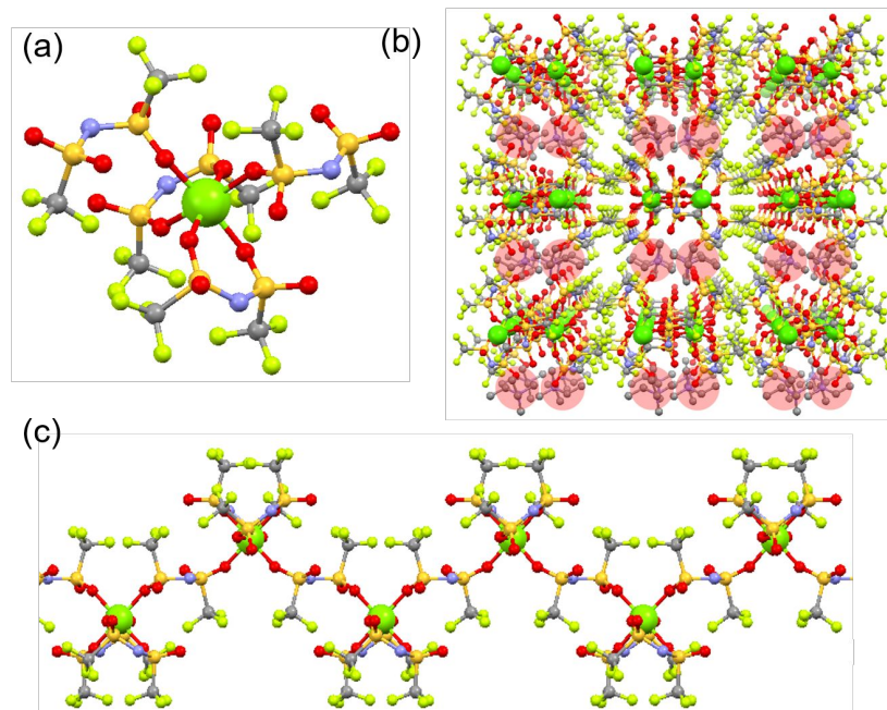
図 2 [N(CH_3)_2(CH_2CH_3)_2][Mg\{N(SO_2CF_3)_2\}_3] の結晶構造解析 (a) マグネシウム周りの構造、(b) マグネシウムイオンと \{N(SO_2CF_3)_2\} アニオンが形成する一次元鎖構造、(c) パッキング図 (薄赤色の部分は N(CH_3)_4 カチオン) (Mg: 緑、C: 灰、O: 赤、N: 青、F: 黄緑、S: 黄、図の簡略化のため水素原子は省略した。)
