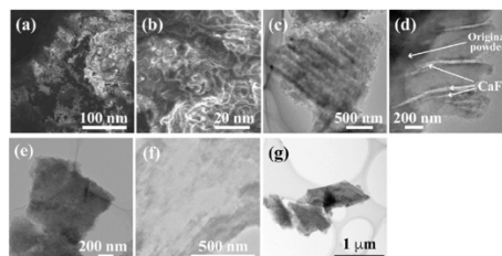
図 8. \text{CaSi}_2 の HF 処理により作製した \text{CaF}_2 ナノシート束の SEM 及び TEM 像 7) .
