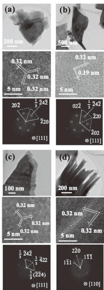
図 6. \text{CaGe}_2 の IP6 処理により作製した (a) 水溶液表面に浮遊, (b) 水溶液中に浮遊, 及び (c) 容器底に堆積した Ge ナノシート剥離片をシート面に垂直な方向から観察した TEM, HRTEM 像及び FFT パターン, (d) 水溶液中に浮遊した剥離片を断面方向に観察した TEM, HRTEM 像及び FFT パターン 5) .
