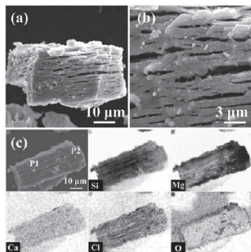
図 4. \text{CaSi}_2 の \text{MgCl}_2 による熱処理により作製した \text{Mg}_2\text{Si}/\text{Si} ナノシート束 コンポジットの SEM, STEM 像及び EDS マッピング 3) .
