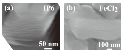
図1. Si基板上に成長させたCaSi 2 よりIP6及びFeCl 2 を用いて作製したSiナノシート束のSEM像 1) 。
