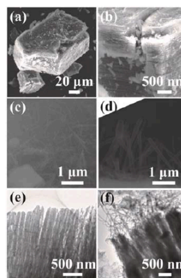
図 5. \text{CaSi}_2 の \text{MnCl}_2/\text{NH}_4\text{Cl} による熱処理により作製した Si 系ナノシート/ナノワイヤ複合体の SEM 及び TEM 像 4) .
