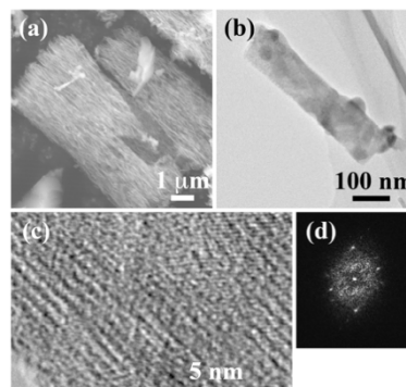
図 9. \text{CaCuSi}_4\text{O}_{10} を HF 及び IP6 処理により作製した酸化物ナノシート束の SEM, TEM, HRTEM 像及び FFT パターン 8) .
