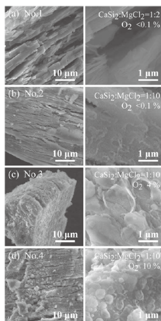
図 7. \text{CaSi}_2 の酸素 (水分) を含む \text{MgCl}_2 雰囲気下における熱処理により作製した \text{Mg}_2\text{SiO}_4 ナノシート束の SEM 像 6) .
