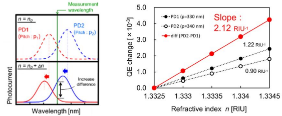
図4. 2フォトダイオード方式における屈折率測定原理(左)と効果(右)。QEはフォトダイオードの量子効率を示す。
