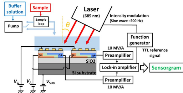
図3. バイオセンシングを行うための測定系
