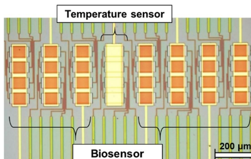
図 2. ワンチップ上に集積化されたバイオセンサーと温度センサー
