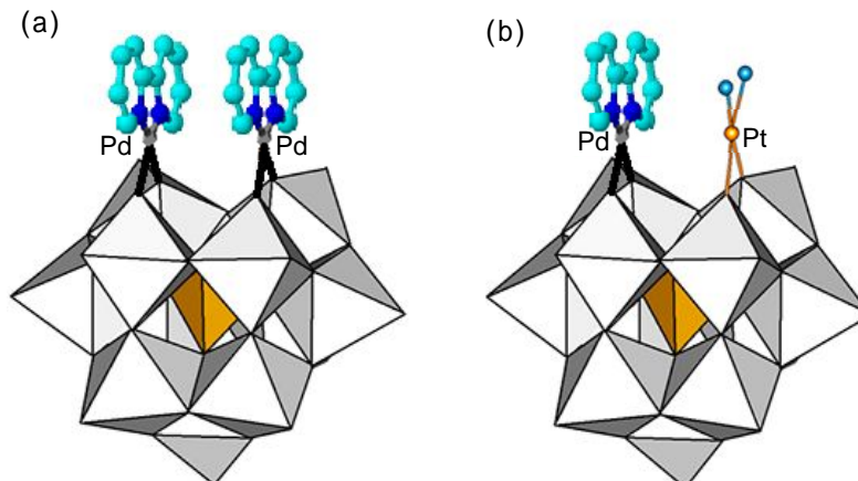
図 6. (a)Pd-2b および (b)Pt-Pd-bimetal の多面体モデル
