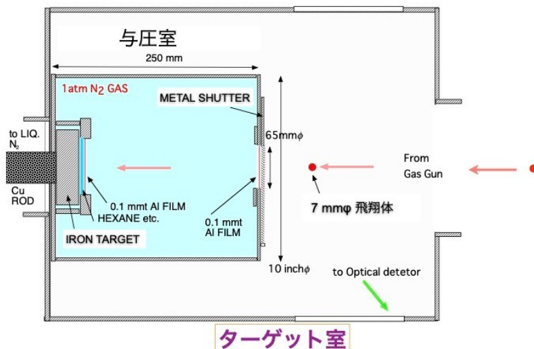
図 2 ガス銃実験装置のターゲット部に置かれた与圧室の模式図。
