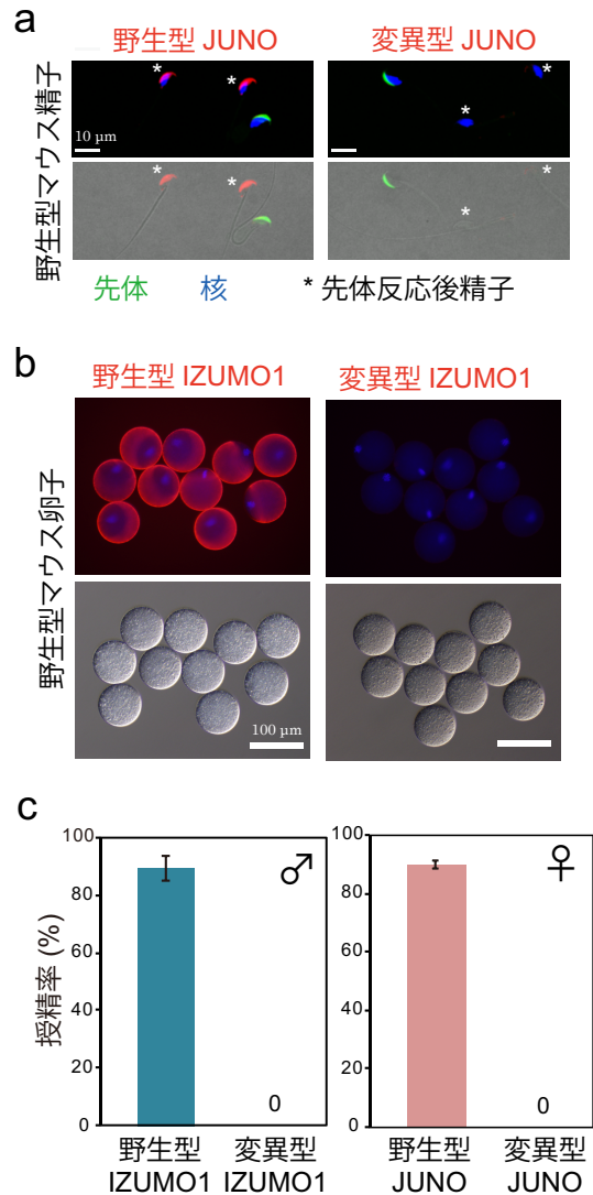
図 3. 変異型 IZUMO1 と変異型 JUNO の解析
