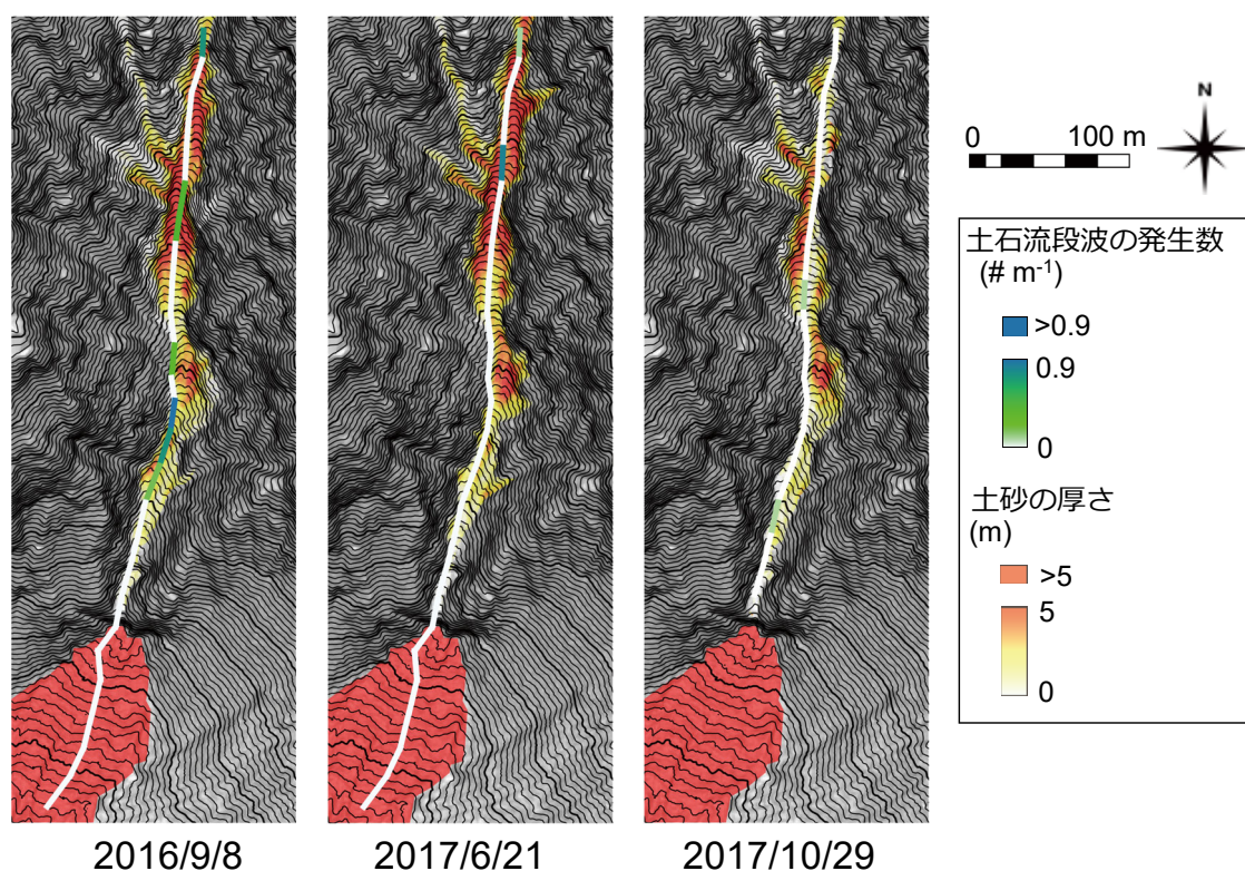
図 静岡県北部大谷崩における土砂貯留マップ (Imaziumi et al., 2019 を一部改変)
