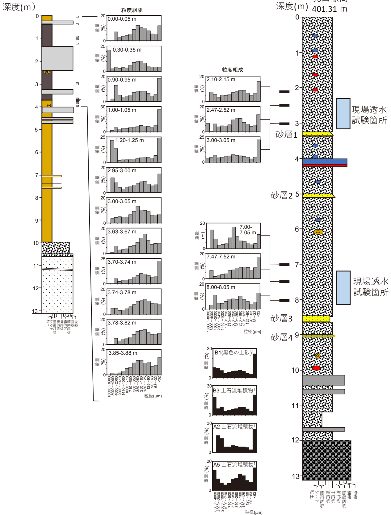
図10 No. 3のボーリングコアの現場透水試験を行った部分の土砂の粒度組成, 地点B1の未崩落の盛土の粒度組成 (北村ほか, 2022a), 砂防堰堤を埋めた土石流堆積物の粒度組成 (北村ほか, 2022d), 集落到達した土石流堆積物の粒度組成 (北村ほか, 2022a).
