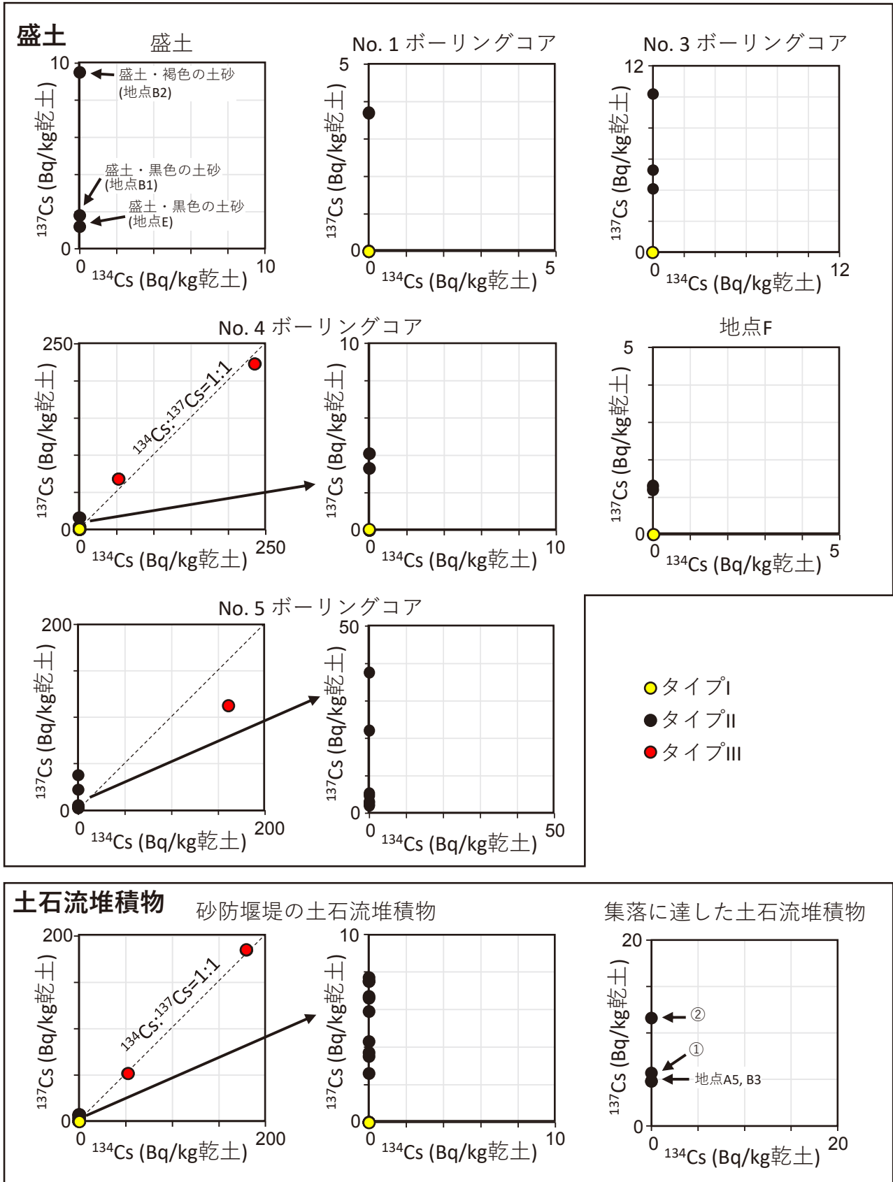
図14 盛土と土石流堆積物の 137 Cs, 134 Csの散布図. 北村ほか (2022c, d) と本研究のデータに基づく.
