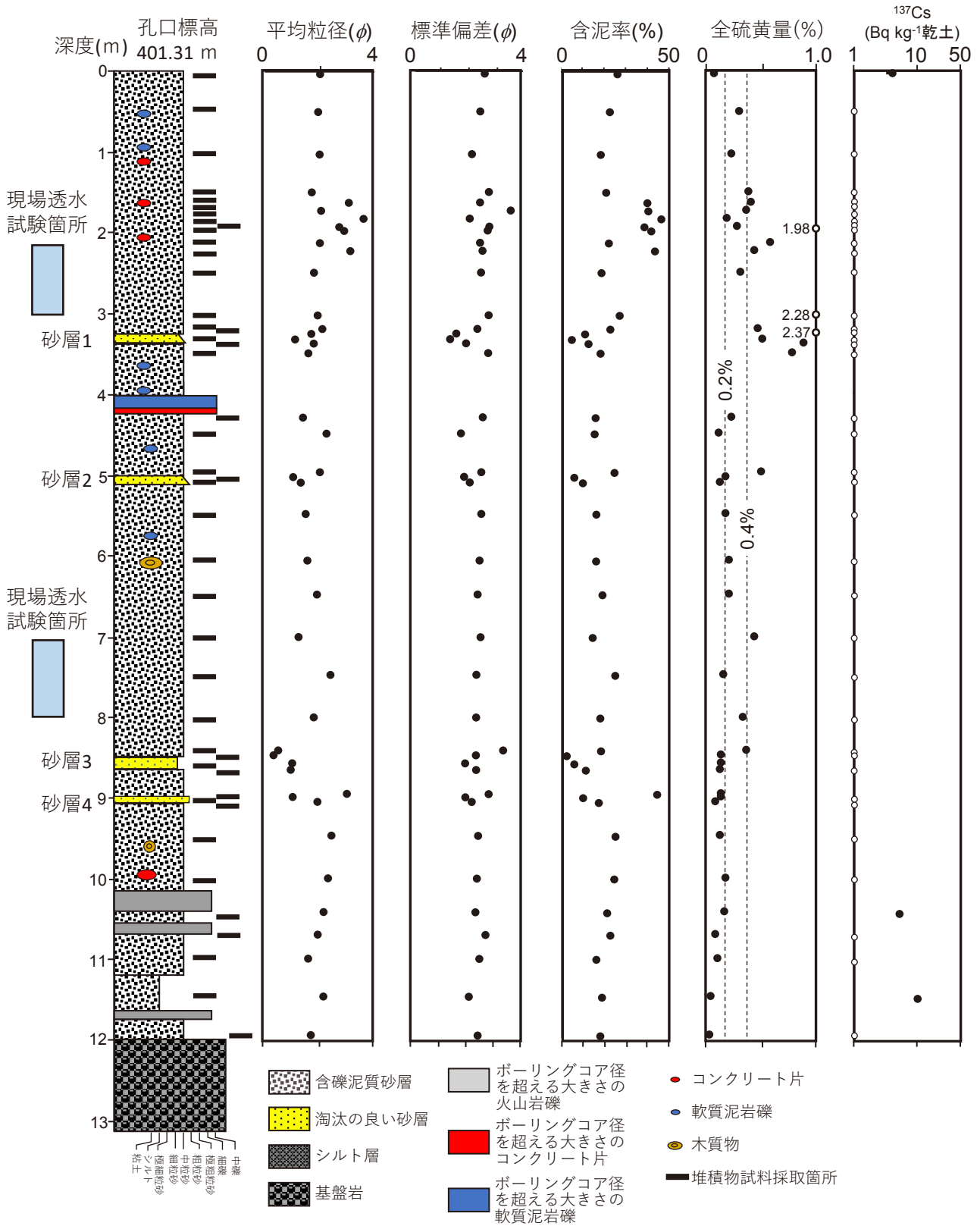
図6 No. 3ボーリングコアの柱状図, 堆積物の平均粒径, 標準偏差, 含泥率, 全硫黄濃度, ^{137}\text{Cs} の層位変化. 放射性セシウム濃度の白丸は検出限界未満を示す.
