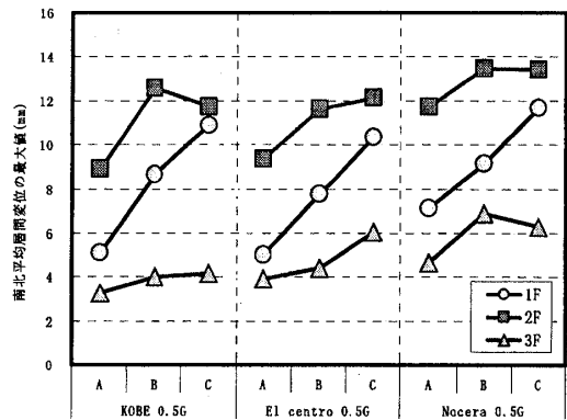
図 4 最大応答比較 (0.5G 入力)
