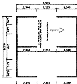
図1 1階平面図 (フェーズB)
