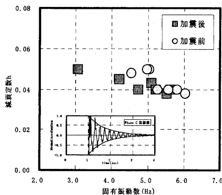
図 3 固有振動数と減衰定数の関係
