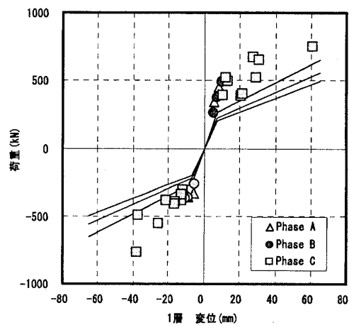
図 5 振動実験による 1 階荷重-応答変位の最大値
