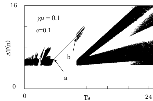
図9 図8にバスの速度変動を加えた場合のバス循環時間と信号サイクルタイムの関係
