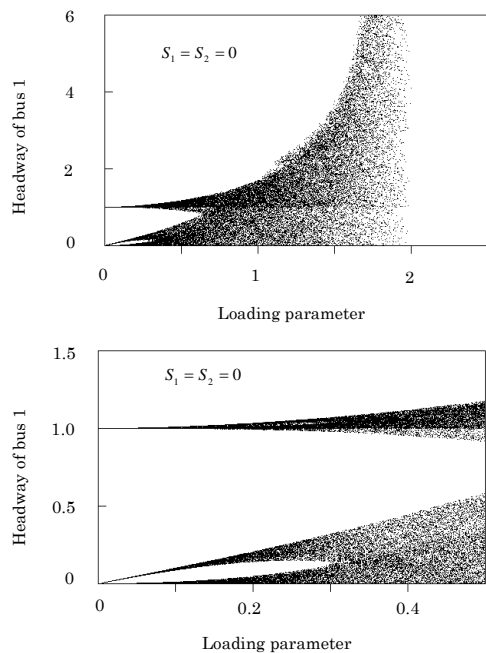
図1 バス1の車間距離とロードパラメータの関係 (スピードアップなし)
