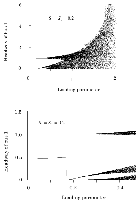
図2 バス1の車間距離とロードパラメータの関係 (スピードアップあり)
