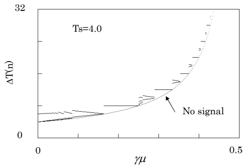
図7 信号サイクルタイムが4.0の場合のバス循環時間とロードパラメータとの関係
