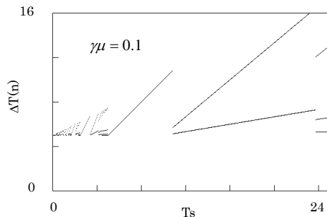
図8 ロードパラメータが0.1の場合のバス循環時間と信号サイクルタイムの関係
