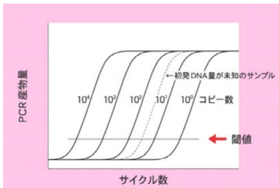
図3 増幅曲線
