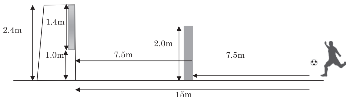
図1 経験者の実験装置
