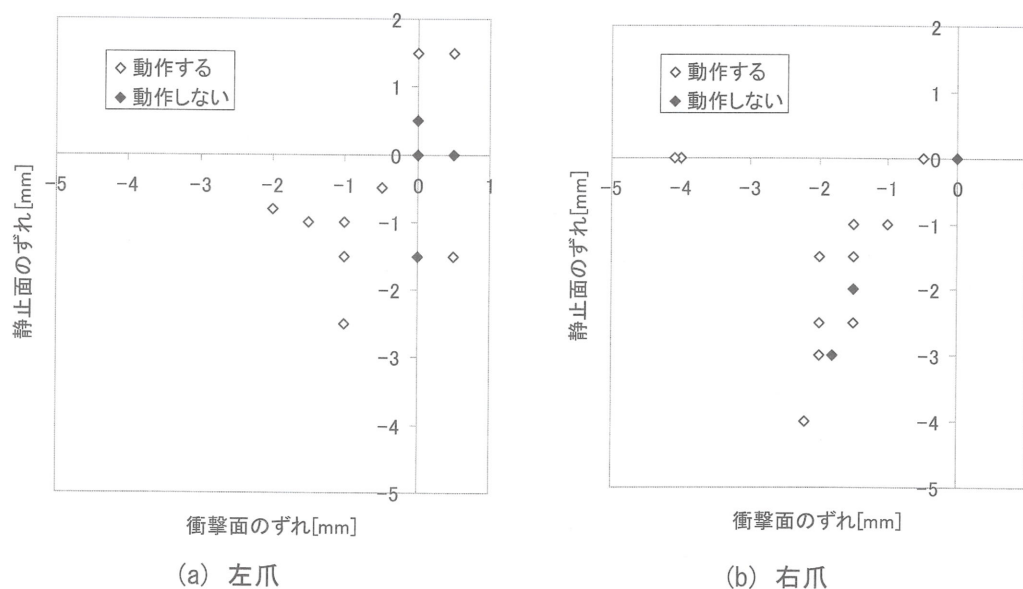
図9 アンクル爪の加工誤差
