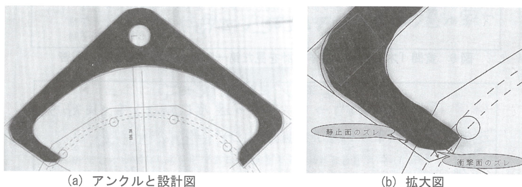
図8 アンクルの加工誤差の測定
