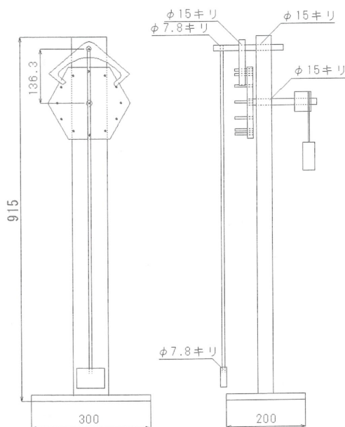
図1 木製機械式振り時計の組み立て図
