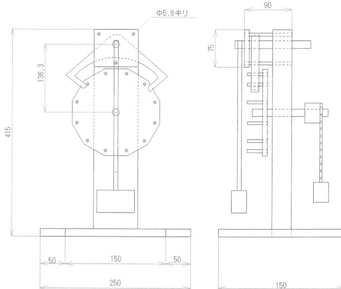
図 10 小型壁掛振り時計の組み立て図
