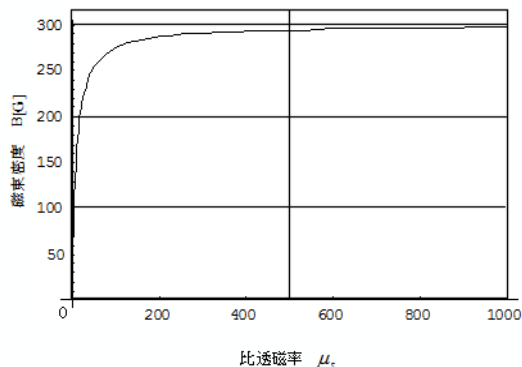
図3 比透磁率と磁束密度の関係
