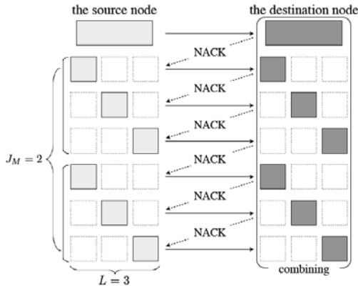
図4 パケット分割を用いた再送制御
