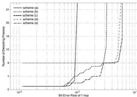
図8 適応中継方式の平均復号回数
