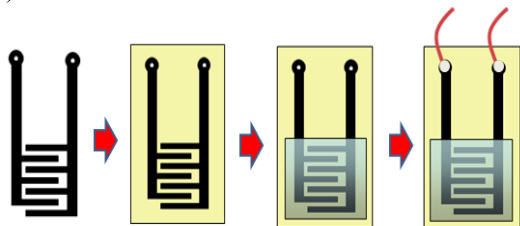
Fig. 1 コプラナー型放電電極の模式図; (a)断面図, (b)作製手順.
