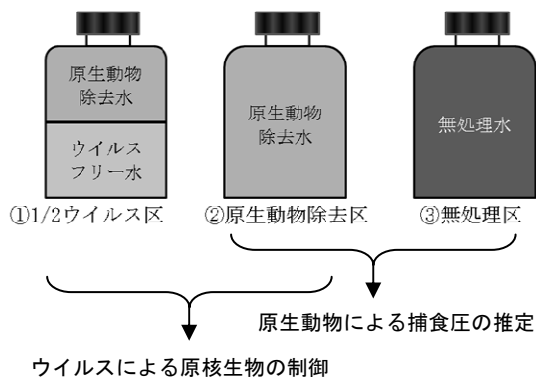
図 1. ウイルスによる原核生物個体群制御実験のスキーム.
