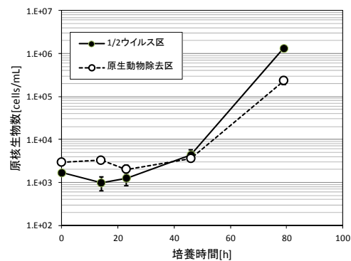
図 2. 北海道幌延 V-140 地下水の分画擬似現場培養実験における原核生物数.
