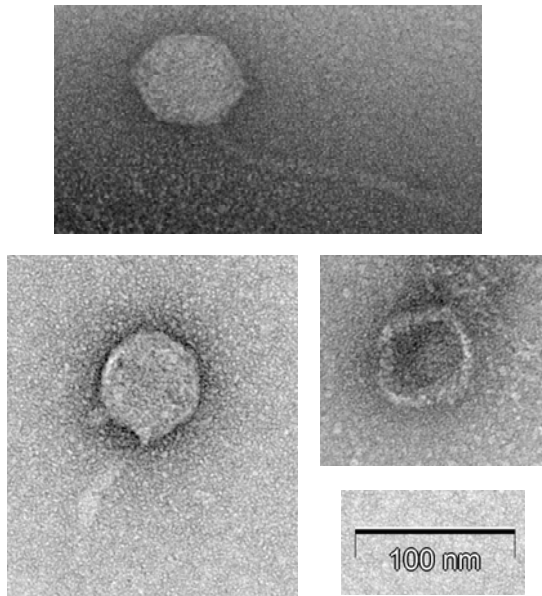
図3. 北海道幌延 V-140 地下水中のウイルス透過型電子顕微鏡写真.
